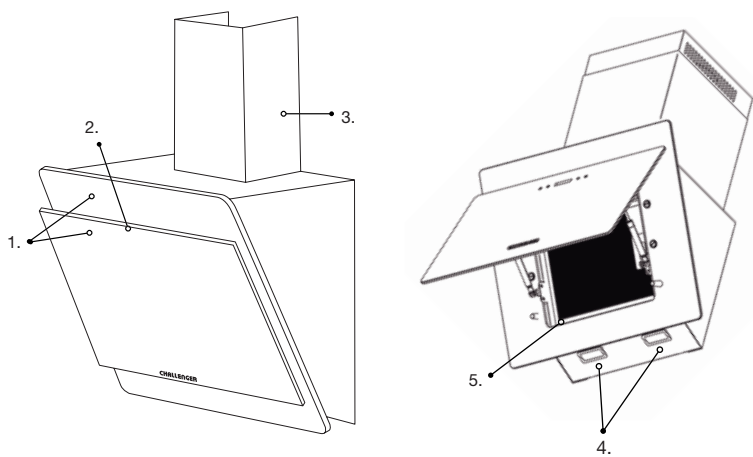
1. Vidrio templado de seguridad. 2. Controles de velocidad de extracción e iluminación. 3. Ducto decorativo. 4. Iluminación tipo LED. 5. Filtros atrapagrasa. 6. Tipo de circulación: Interna / Externa.
